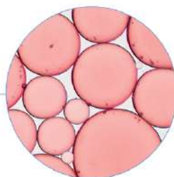
Kyselina laktobionová 20%
