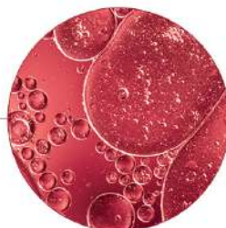
Kyselina pyrolidonkarboxylová
