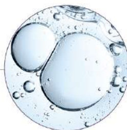
Kyselina lipoová
