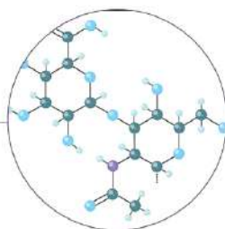
Kyselina hyaluronová
